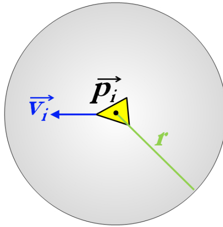
Figura 7.4: La figura muestra la posición que representa las coordenadas donde está ubicado el cuerpo del boi d. La velocidad determina el desplazamiento del boi d. El área de percepción está determinada por un radio.
