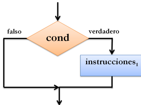
Figura 4.4: Diagrama de flujo que muestra el funcionamiento de la estructura de decisión simple.
