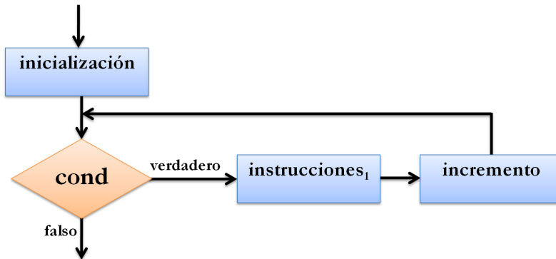
Figura 4.9: Diagrama de flujo que muestra el funcionamiento de la estructura repetir para .
