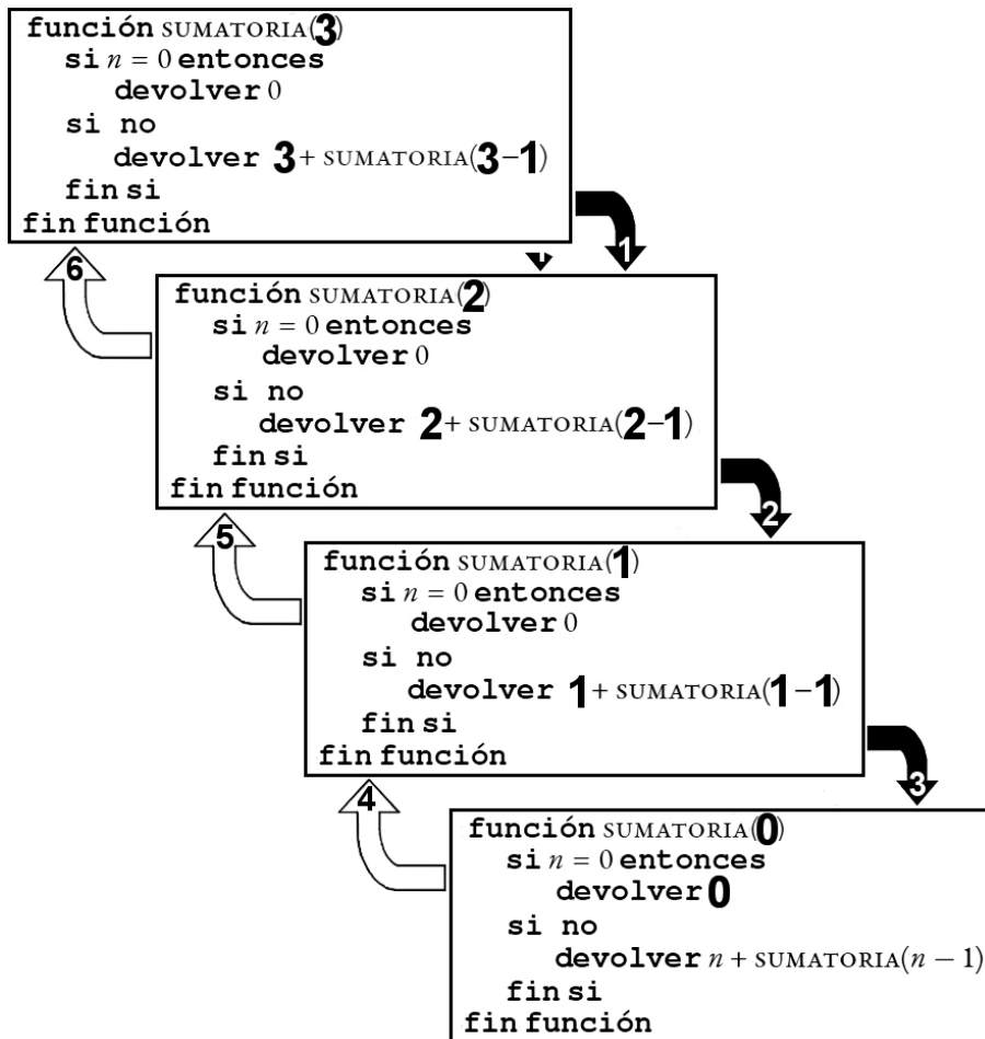
Figura 5.8: Copias recursivas. Los encabezados de los procedimientos muestran el valor del parámetro n . Las flechas negras muestran la “delegación” en otra copia del procedimiento (es decir, una invocación recursiva). Las flechas blancas indican la devolución del control al procedimiento que invocó la copia recursiva.
