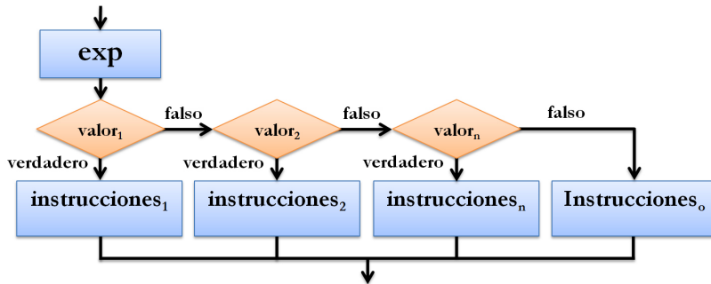
Figura 4.6: Diagrama de flujo que muestra el funcionamiento de la estructura de decisión múltiple.
