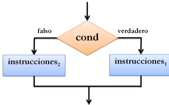
Figura 4.5: Diagrama de flujo que muestra el funcionamiento de la estructura de decisión disyuntiva.
