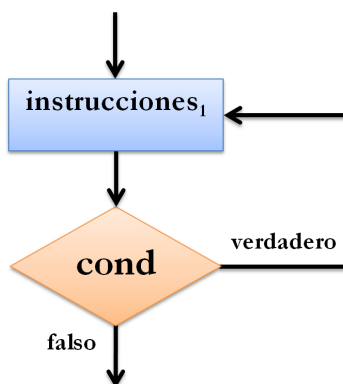
Figura 4.8: Diagrama de flujo que muestra el funcionamiento de la estructura repetir hasta .
