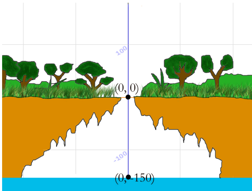
Figura 7.2: Representación esquemática del problema de caída libre.
